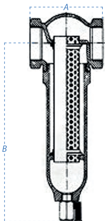
Type C og R Gjenget innv.
