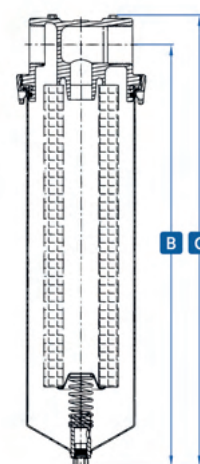
Dimensjoner (mm)
